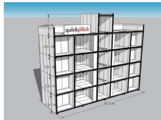
Arquitectura y modulación de edificios industrializados
